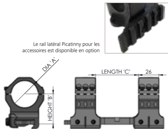
A = diamètre du collier / B = hauteur / C = distance entre les colliers
